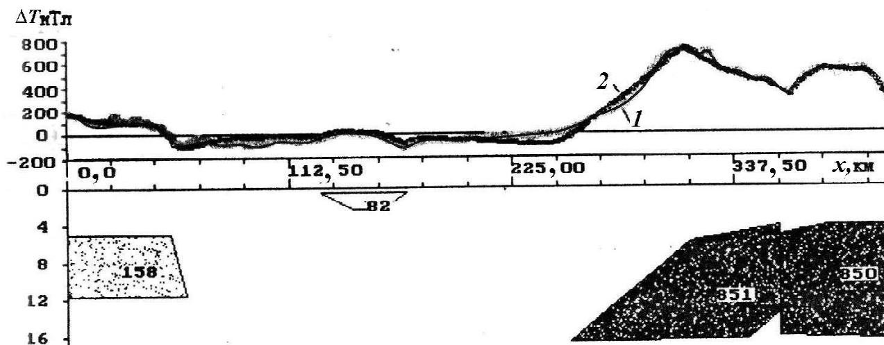
Рис. 3. Аномальное магнитное поле и результаты формального автоматизированного подбора параметров магнитовозмущающих источников вдоль галса 0404. Условные обозначения см. на рис. 2.
