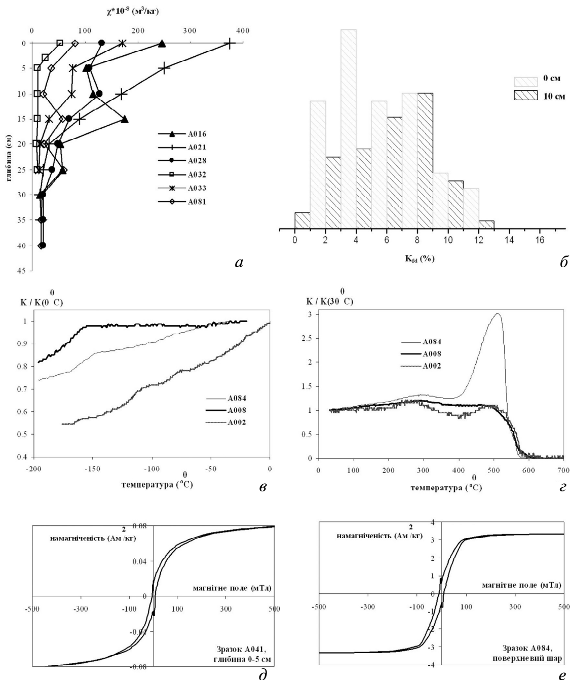
Рис. 2. Петромагнітні властивості ґрунтів Північної Астурії (пункти A008, A016, A021, A081, A084 розташовані в зонах впливу промислових підприємств, пункти A002, A032, A033, A041 – фонові)
