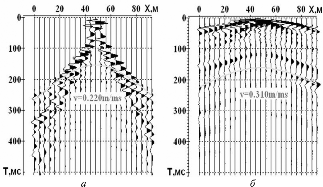
Рис. 2. Кинематика отраженных SH -волн: a — нормальный скоростной разрез (лето), b — инверсионный скоростной разрез (зима)
