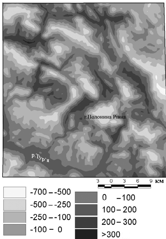
Рис. 6. Різниця висот умовної топографічної поверхні (в м) у просторовому зрізі 15 км та реальної топоповерхні
