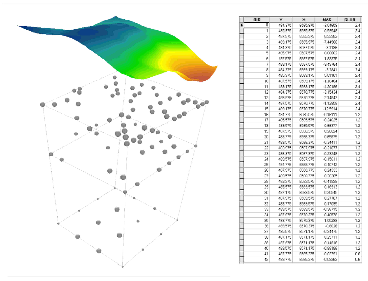
Рис. 2. Аппроксимационная конструкция и структура таблицы содержания shp -файла сеточной модели
