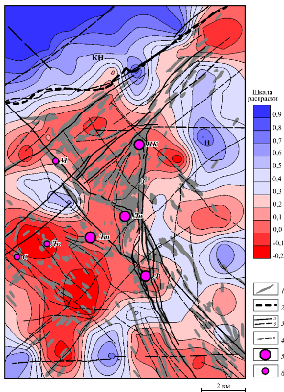
Рис. 4. Схематическая карта распределения коэффициента парной корреляции Пирсона плотности и магнитной восприимчивости пород на поверхности кристаллического фундамента в районе Новоконстантиновского рудного поля: 1 – микроклин-альбитовые метасоматиты и альбититы (формация щелочных натриевых метасоматитов зон глубинных разломов PR_1^{mt} ); 2 – граница между Новоукраинским массивом (Н) и Корсунь-Новомиргородским плутоном (КН); 3 – главные разломы: а – достоверные, б – предполагаемые; 4 – второстепенные разломы; 5 – месторождения урана (НК – Новоконстантиновское, Лн – Лесное, Д – Докучаевское, Лт – Летнее); 6 – рудопроявления урана (М – Мануйловское, З – Залесное, Дк – Декабрьское, С – Степное)
