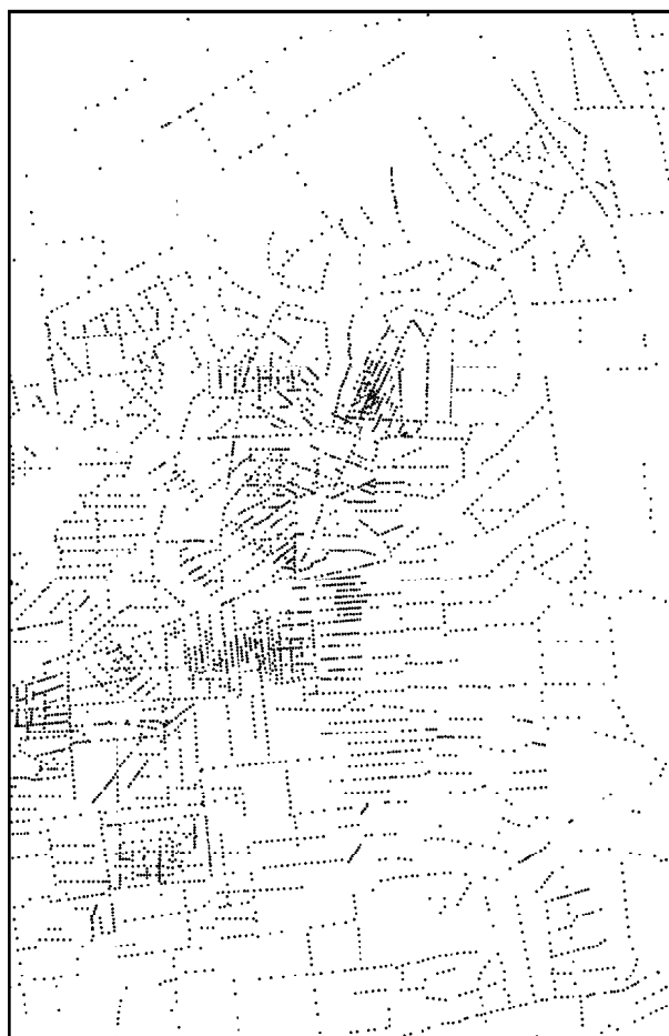
Рис. 2. Схема расположения скважин (чёрные точки) на площади Новоко́нстанти́новского рудного поля (по данным КП “Кировгеология”)
