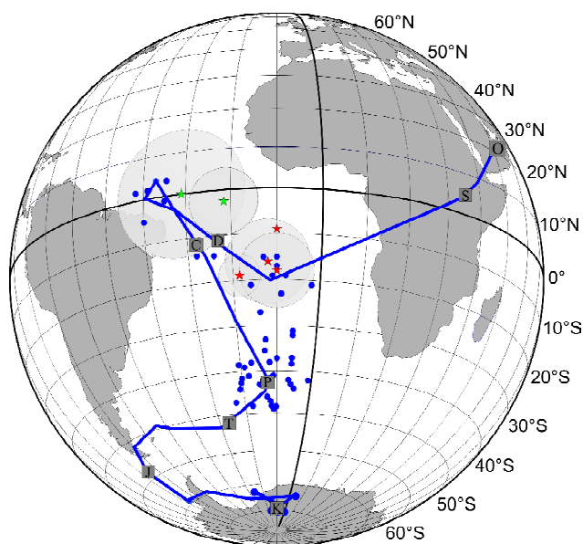
Рис. 2. Траектория кажущейся миграции полюса для Балтики (ВЕП) в фанерозое. Синие точки — ключевые палеомагнитные полюса, на основании которых построена кривая [14]; красные звездочки — силурийские полюса (с радиусом круга доверия при 95%-й вероятности для среднего направления), полученные авторами данной работы [1, 10]; зеленые звездочки — девонские полюса, полученные авторами данной работы [2, 5]; квадраты с латинскими буквами — начало геологического периода
