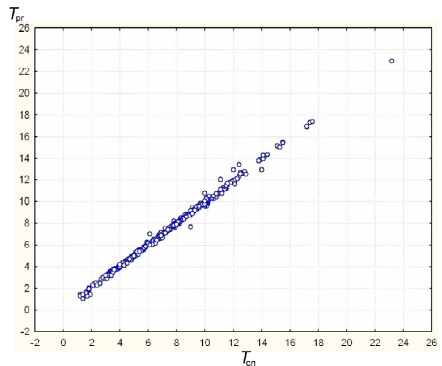
Рис. 3. Співвідношення часів, указаних у сейсмологічному бюлетені, та часів, прогнозованих за нейронною мережею
