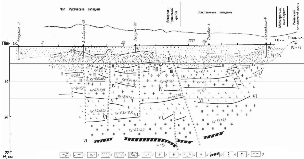
Рис. 1. Сейсмогеологічний розріз земної кори вздовж Закарпатського прогину: 1 – заломлювальні горизонти із зазначеними граничними швидкостями ( V ); 2 – відбивні горизонти (I–VII); 3 – пластова швидкість, км/с; 4 – неогенова моласа; 5 – вулканіти в осадовому чохлі; 6 – мезозойсько-палеогенова складчаста основа прогину; 7 – палеозойський (?) метаморфізований фундамент; 8 – шар пониженої швидкості всередині “гранітного” шару; 9 – докембрійський (?) кристалічний комплекс; 10 – “базальтовий” шар; 11 – шар пониженої швидкості в основі земної кори; 12 – поділ Мохоровичича; 13 – розломи; 14 – бурова свердловина; 15 – крива \Delta g
