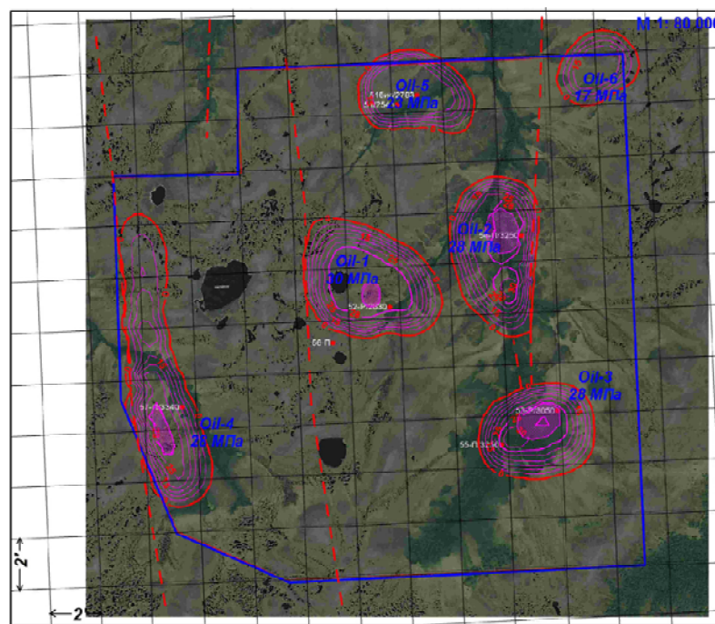
Рис. 5. Карта аномальных зон типа “запасы углеводородов” на Восточно-Вуемском лицензионном участке (Россия) на спутниковом снимке местности, по результатам частотно-резонансной обработки данных ДЗЗ. Условные обозначения см. на рис. 4
