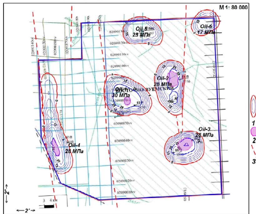
Рис. 4. Карта аномальных зон типа “запасы углеводородов” на Восточно-Вуемском лицензионном участке (Россия) на карте-схеме расположения сейсмических профилей и пробуренных скважин, по результатам частотно-резонансной обработки данных ДЗЗ: 1 – изолинии максимальных значений пластового давления флюидов в коллекторах, МПа (комплексный параметр); 2 – “газовая шапка”; 3 – тектоническое нарушение
