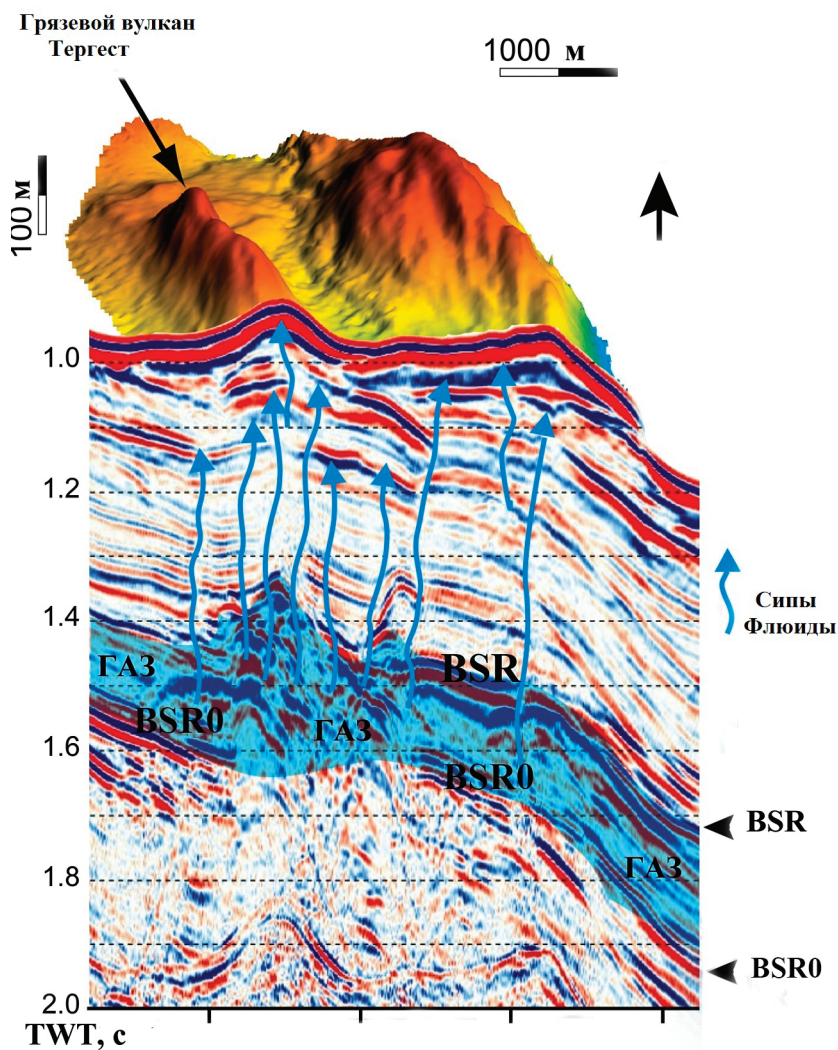
Рис. 4. Схематический разрез вдоль профиля через зону грязевого вулкана Тергест в море Росса, по [6]. Показаны глубинные границы BSR и BSR0, фиксирующие положение ЗГО в разрезе. Положение профиля показано на рис. 1
