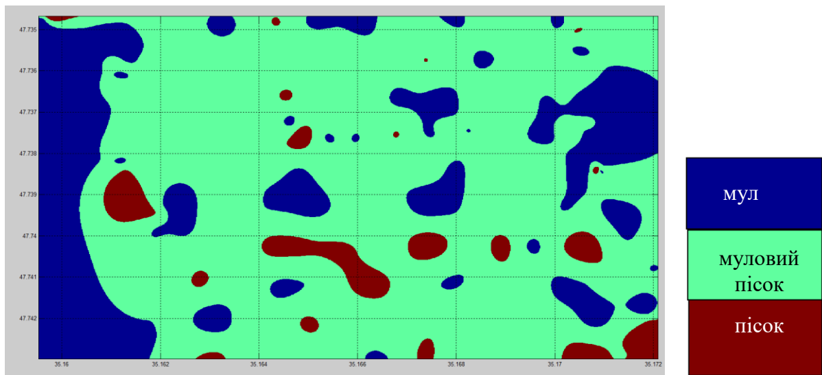
Рис. 7. Стратифікація верхнього шару донних відкладів обстеженого полігону
