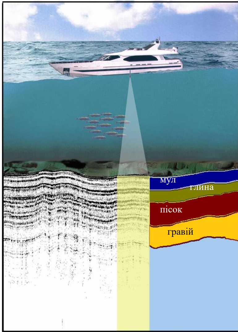
Рис. 1. Принцип роботи гідроакустичного профілографу
