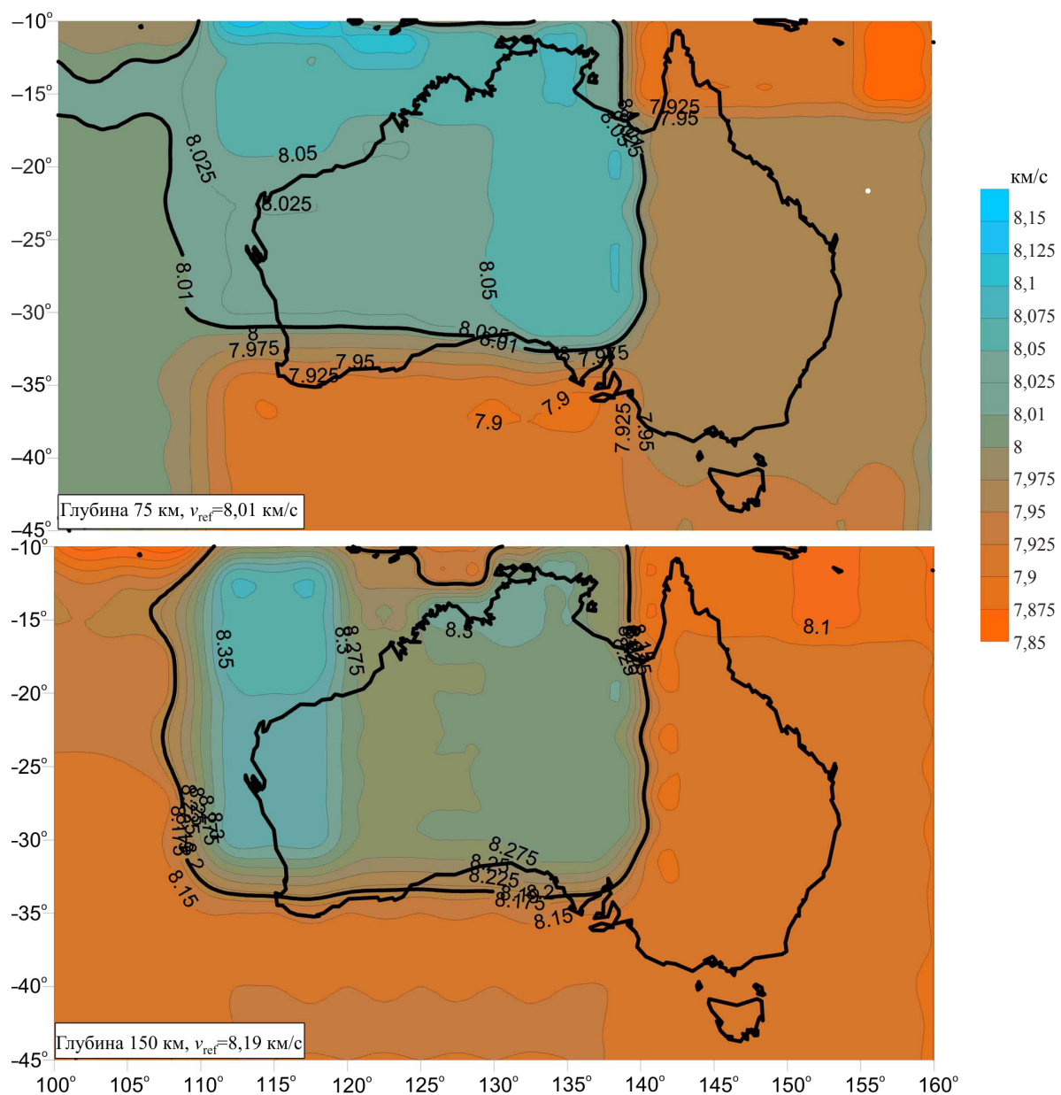
Рис. 4. Горизонтальные сечения трехмерной P -скоростной модели мантии Австралии на глубинах 75 и 150 км
