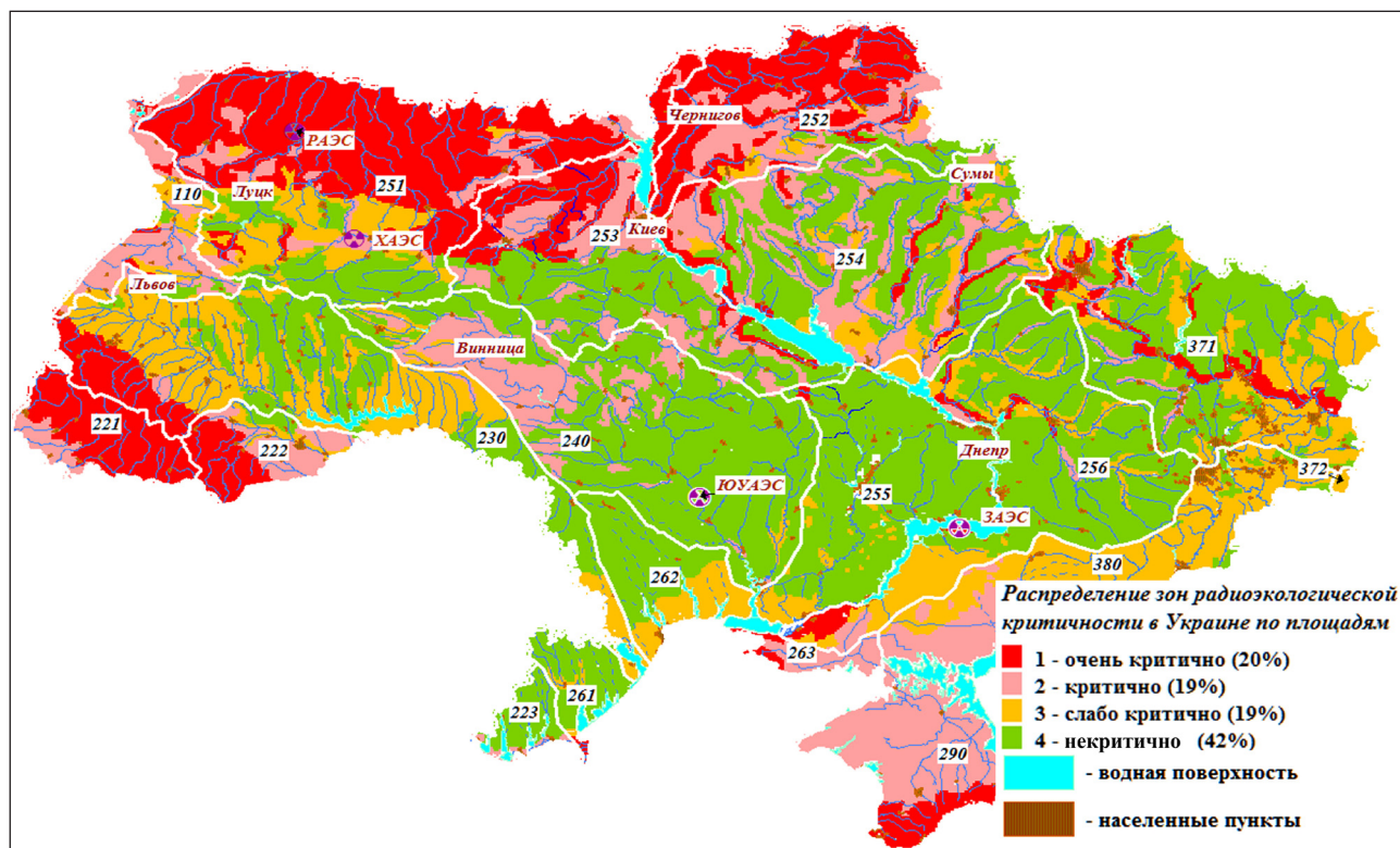
Рис. 3. Распределение зон радиоэкологической критичности по гидрографическим районам территории Украины
