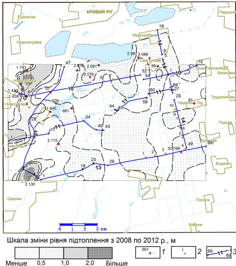
Рис. 3. Прогнозна карта складової "підтоплення" у рівні підземних вод за період 2008–2012 рр.: 1 – точка, в якій визначено рівень підземних вод і номер свердловини або колодязя; 2 – свердловина інтерпретаційного буріння та її номер; 3 – профіль ВЕЗ та його номер, номери кінцевих точок на профілі
