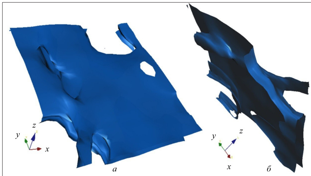
Рис. 1. 3D зображення зміни значень уявного електричного опору за період з 2008 по 2012 рр.: вигляд зверху з південно-західного кута площі досліджень (а) та знизу (б)
