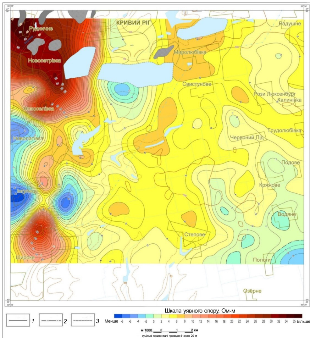
Рис. 5. Карта зміни значень уявного опору за проміжок часу з 1983 по 2008 р. Ізолінії: 1 – додатних змін значень уявного опору, 2 – нульових, 3 – від’ємних
