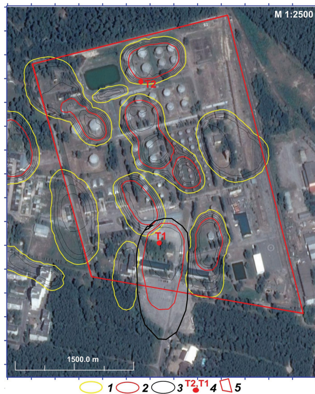
Рис. 8. Карта геоэлектрических аномальных зон типа "техногенная залежь топлива" на спутниковом снимке территории нефтебазы (по данным частотно-резонансного дешифрирования спутниковых снимков). Резонансные частоты пробы 2: 1 – контуры аномальных зон; 2 – наиболее перспективные поисковые зоны; 3 – контур аномальной зоны по резонансным частотам пробы 1; 4 – скважины отбора образцов топлива; 5 – границы нефтебазы
