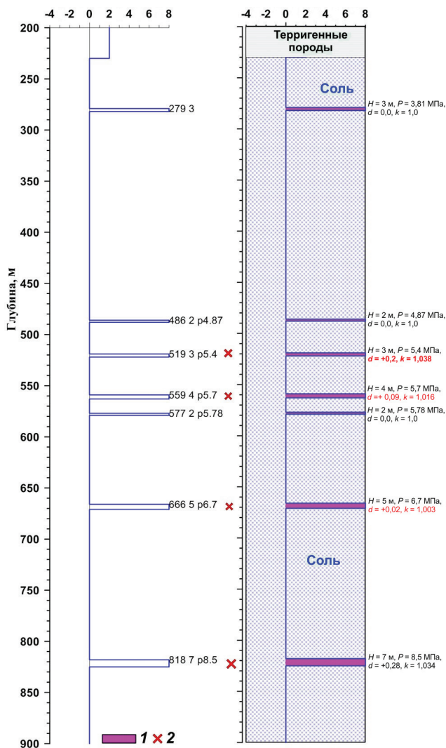
Рис. 7. Результаты вертикального сканирования аномальной зоны типа "газ" в районе емкости 3Е: 1 – прогнозируемый газ в пропластках брекчии; 2 – наиболее газосодержащие пласты; H – мощность пластов; P – пластовое давление; d – разность между пластовым и гидростатическим давлениями; k – отношение пластового давления к гидростатическому
