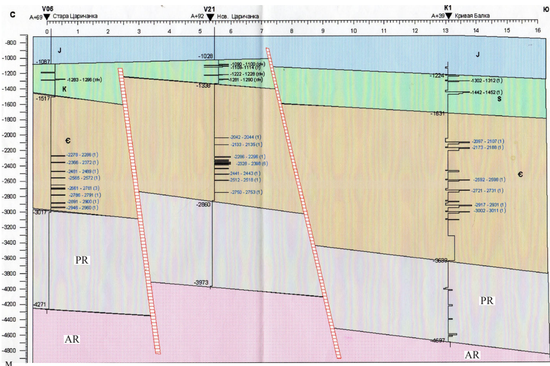
Рис. 7. Успеновская площадь. Схематические геоэлектрические разрезы западной (а) и восточной (б) частей площади. Вертикальная шкала глубин дана в абсолютных значениях
