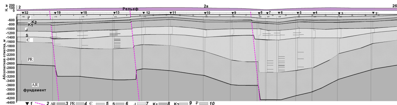
Рис. 4. Успеновская площадь. Схематический структурно-геологический разрез вдоль профиля 2–2а–2б через геоэлектрические аномалии по данным зондирования ВЭРЗ: 1 – точки зондирования; 2 – зоны тектонических нарушений; 3 – граниты; 4 – черные сланцы; 5 – аргиллиты, алевролиты, песчаники; 6 – органогенные известняки; 7 – глины; 8 – песчаники; 9 – мел; 10 – глины
