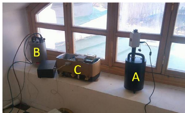
Рис. 4. Зовнішній вигляд сейсμοприймачів для вимірювання зміщення, швидкості та прискорення поширення коливань: А – акселерометр; В – велосиметр; С – лазерний вимірювач вертикальних зміщень
