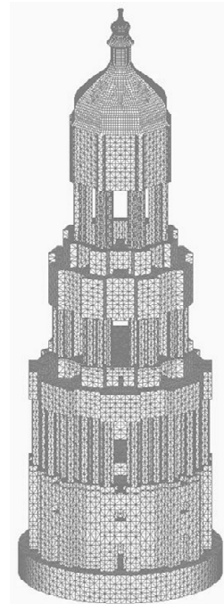
Рис. 2. Розрахункова модель
