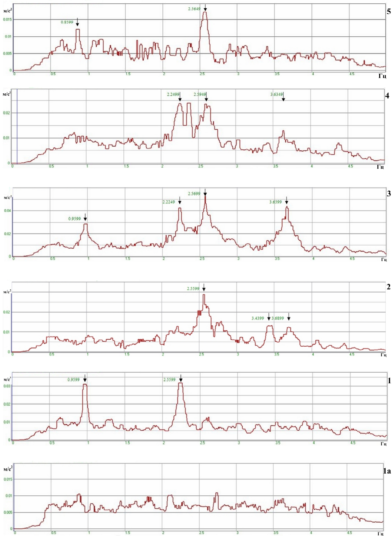
Рис. 6. Розподіл піків основних частот за їх максимальним значенням для N-компоненти (північ–південь) прискорення мікросейсмічних коливань залежно від висоти точки вимірювання (відповідно до рис. 5 зверху вниз точки 5–1а)
