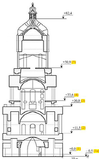
Рис. 5. Схема розміщення сейсмодатчиків за висотою дзвіниці
