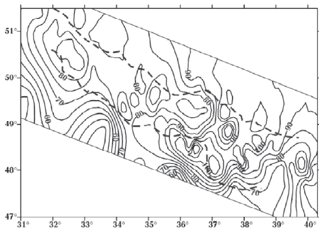
Рис. 1. Карта розподілу температур (°C) у регіоні Дніпровсько-Донецької западини на глибині 3000 м [15]
