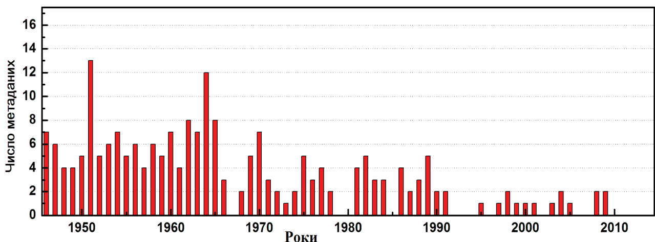
Рис. 5. Часовий розподіл метаданих
