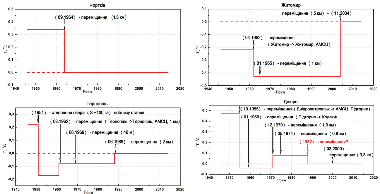
Рис. 17. “Станційні сигнали” у річних рядах деяких станцій (стрілками вказано метадані) Fig. 17. “Station signals” in annual series of some stations (arrows indicate metadata)
