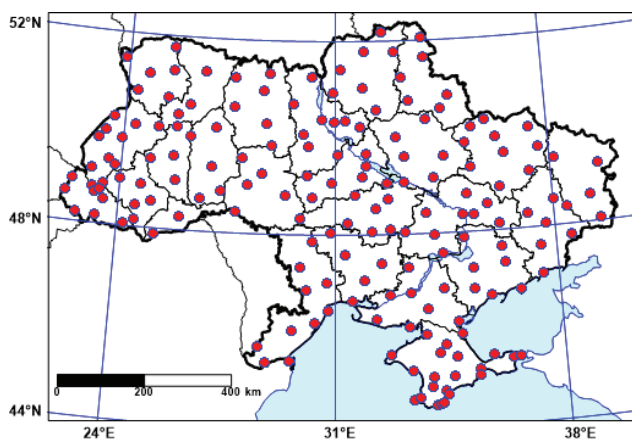
Рис. 3. Просторовий розподіл метеорологічних станцій, дані яких використано для гомогенізації (для створення гомогеної БД)
