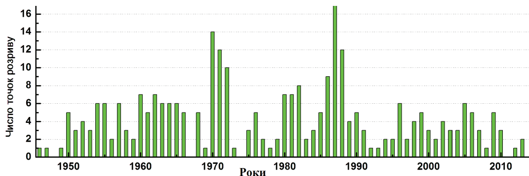
Рис. 14. Часовий розподіл ідентифікованих точок розриву Fig. 14. Time distribution of the identified break points
