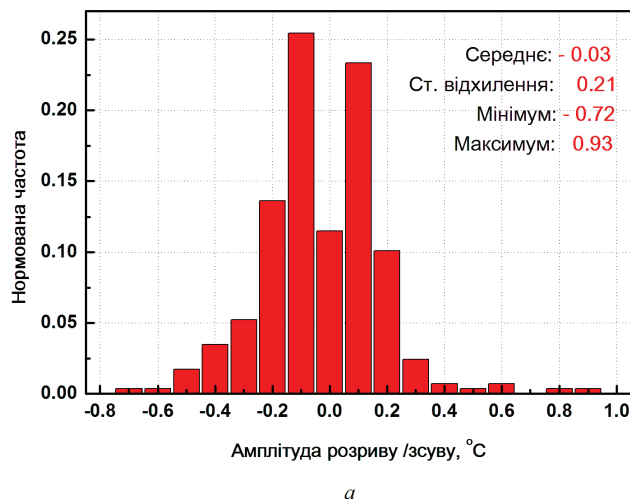
Рис. 16. Розподіл амплітуд (а) і факторів (б) виявлених зсувів/розривів у річних рядах
