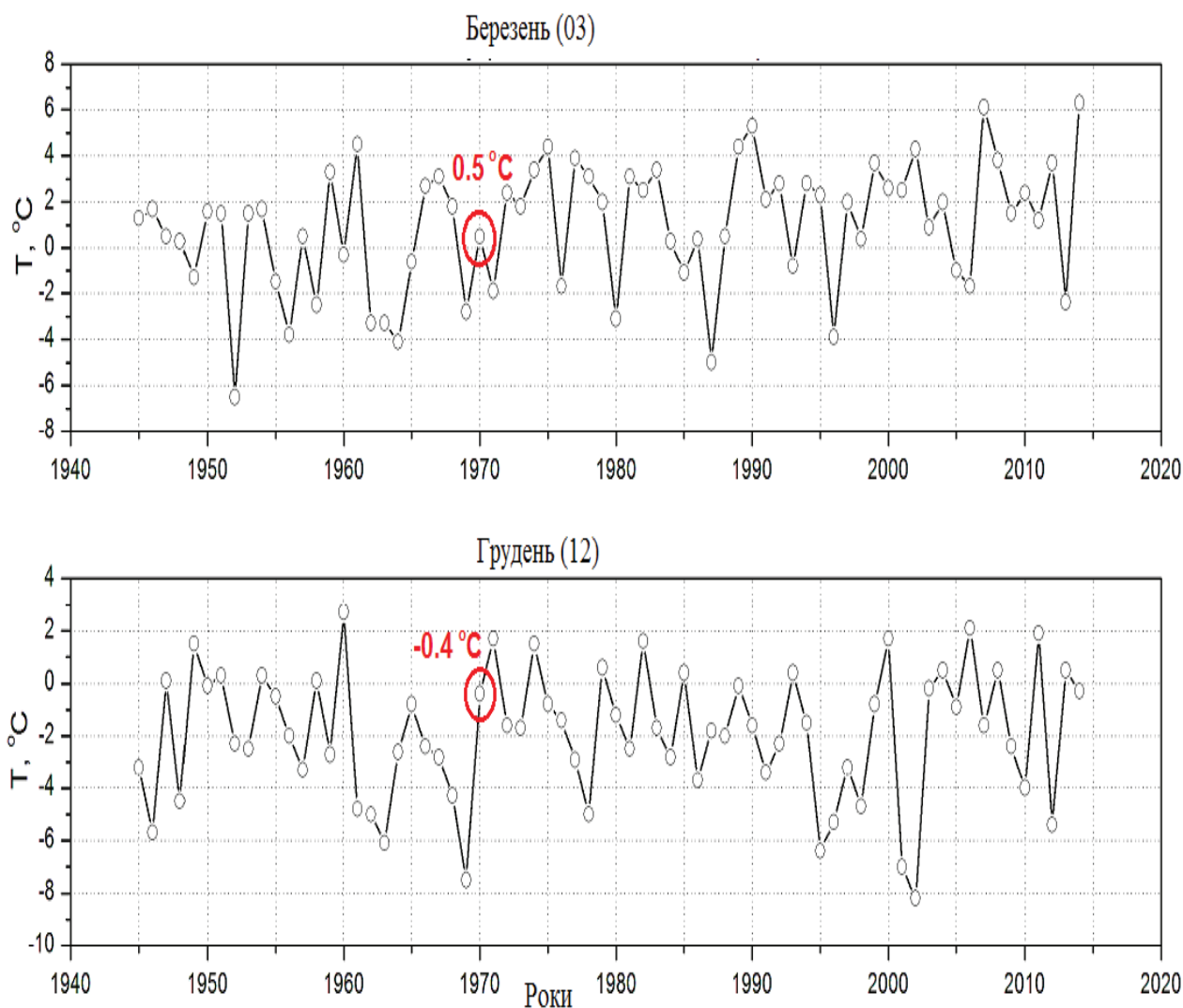
Рис. 8. Виправлені ряди даних на станції Луцьк для березня (03) та грудня (12)
