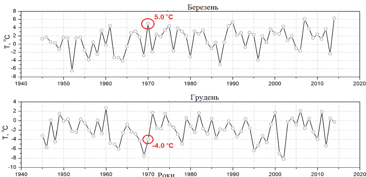
Рис. 6. Первинні (не гомогенізовані) ряди даних на станції Луцьк для березня та грудня
