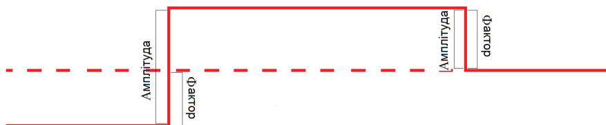
Рис. 15. Типовий “станційний сигнал” та його характеристики (амплітуди/фактори), які розраховує програма HOMER
