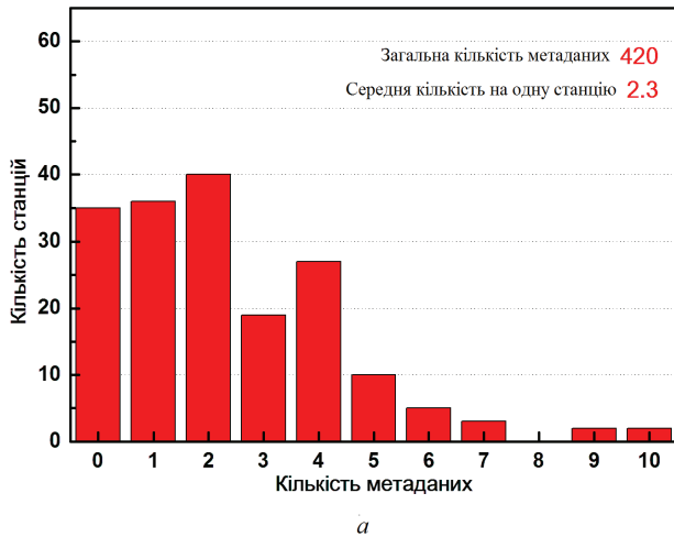
Рис. 4. Розподіл кількості станцій за кількістю метаданих (в основному — переміщень станцій: а — від початку роботи станцій; б — для періоду 1946—2014 рр.
