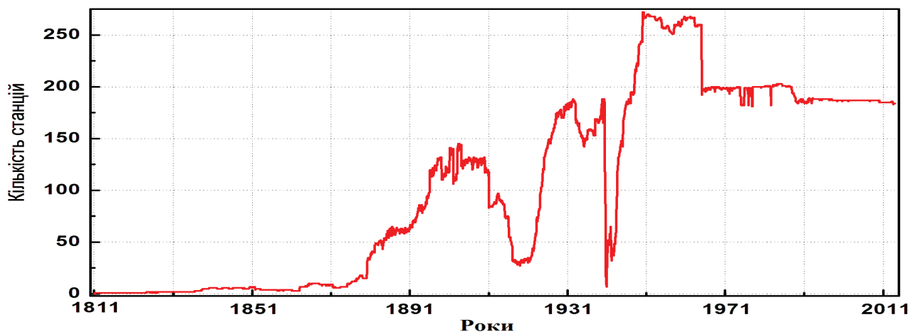
Рис. 1. Еволюція загальної кількості метеорологічних станцій, які працювали на території України протягом періоду 1812–2014 рр.
